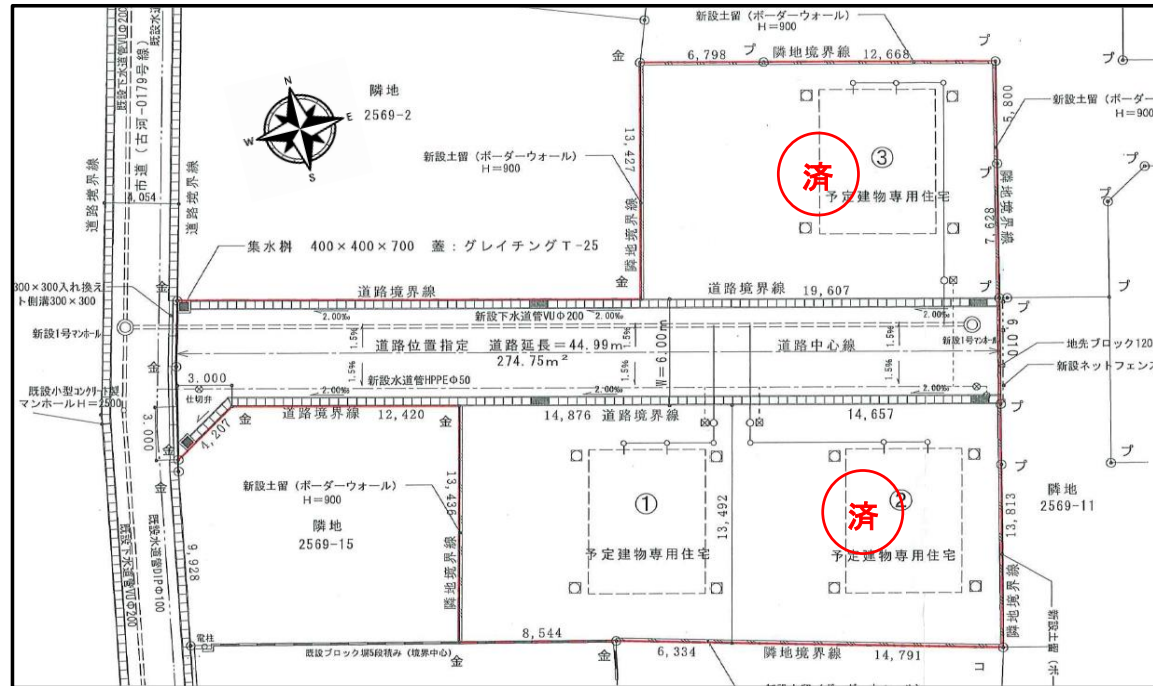
区画割図
