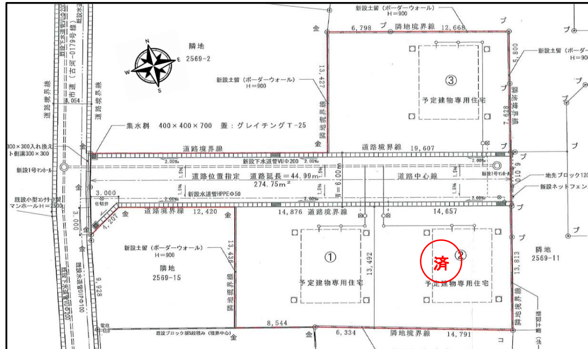
区画割図
